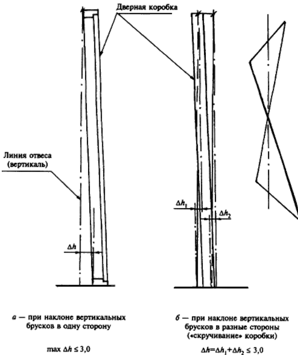
Рисунок В.2 - Определение отклонений дверной коробки
