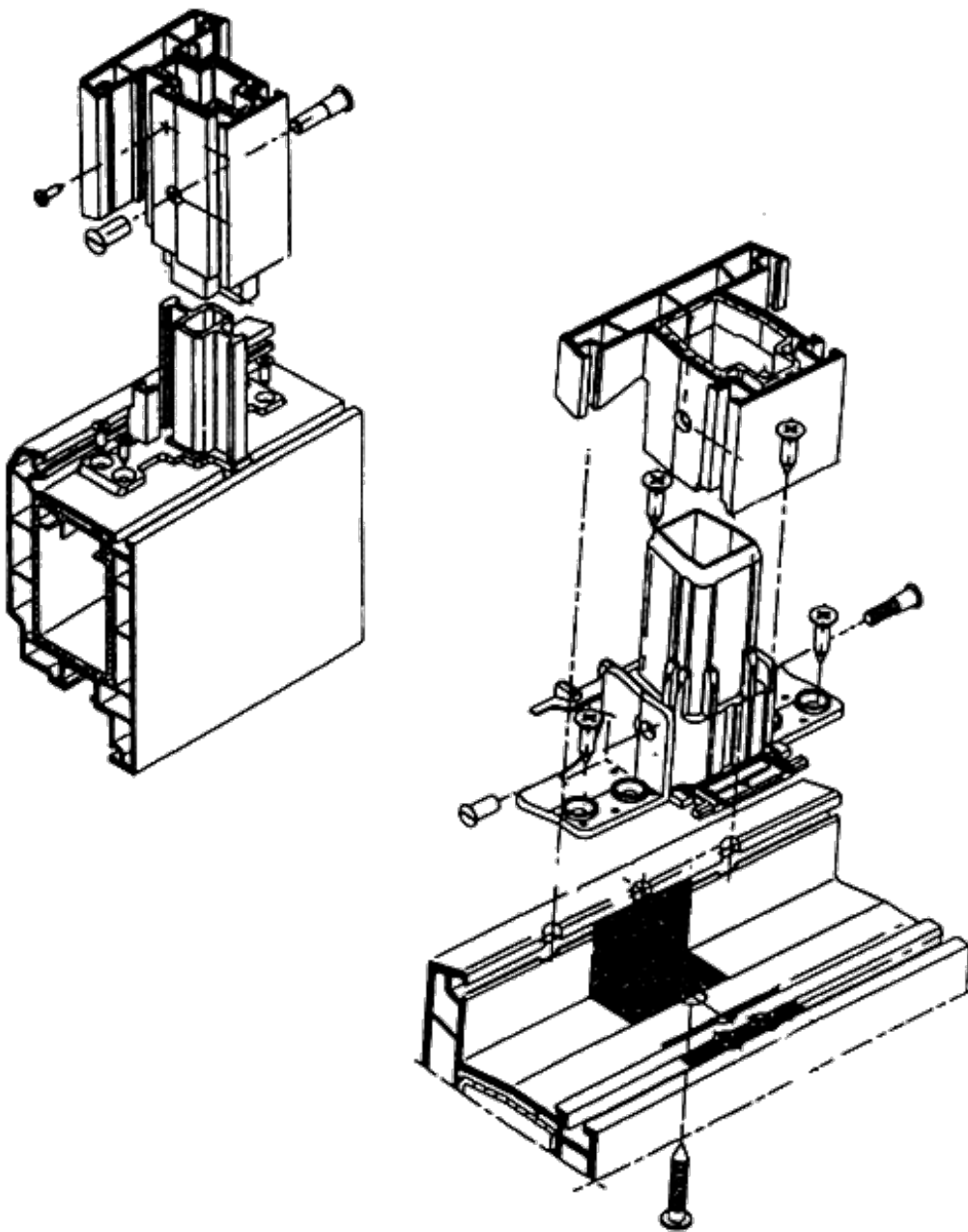
Рисунок 9 - Примеры крепления импостов (механическое соединение)
