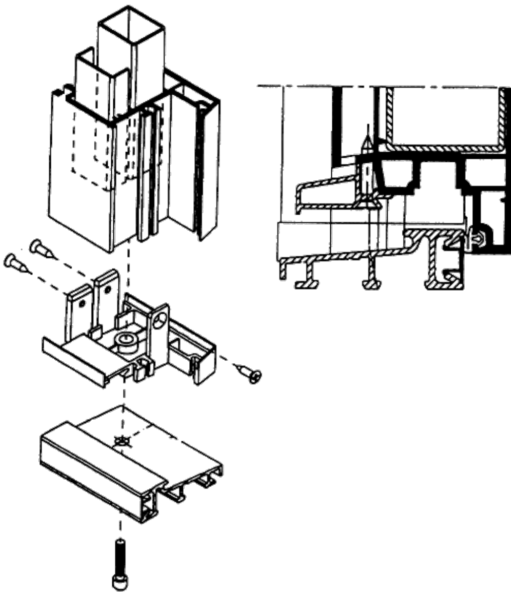
Рисунок 10 - Пример крепления порога (механическое соединение)
